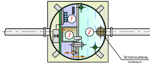
Разрез А-А (1:10)
